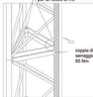
vista prospettica fissaggio traliccio-traliccio
